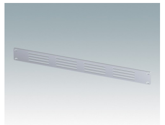
M6019011 Plaque avant 1Ux19" avec aération Aluminium Anodisé mat 482,6x3x43,6mm
