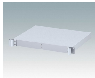
M6219125 COMBIMET 19" 1Ux365mm panneau supérieur plein Aluminium Gris clair RAL 7035 43,6x482,6x365mm
